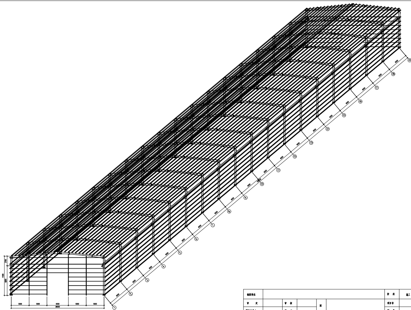
钢架轴测图 1:100
