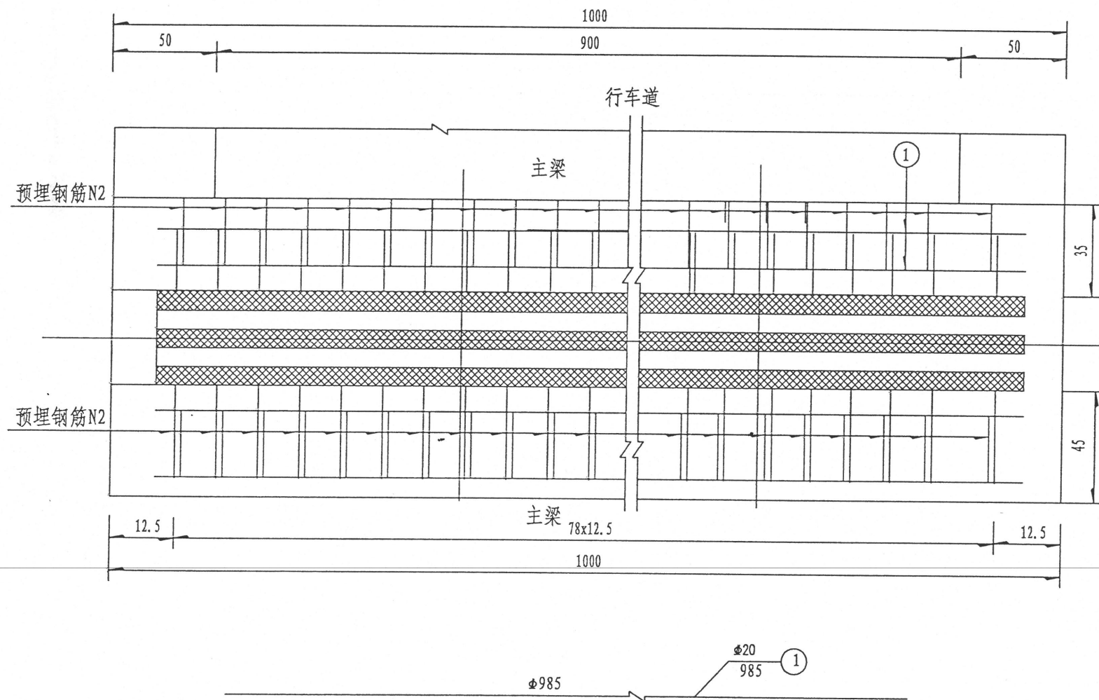
平面
