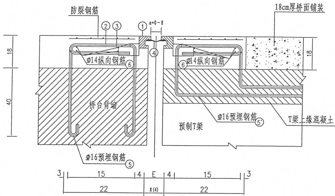
伸缩缝立面示意图
