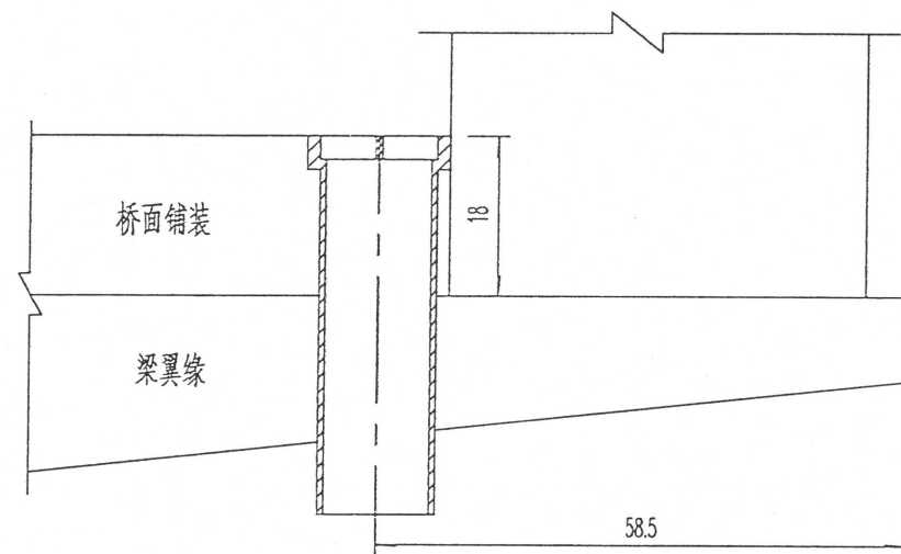
安装示意图
