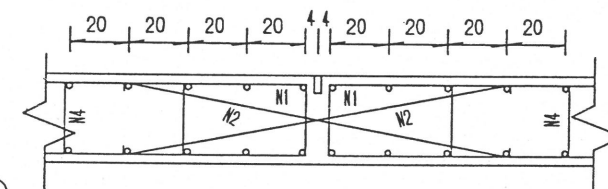
A大样 1:25
